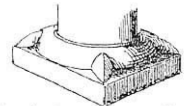
Base de piles ronde avec griffes G. Boulangé (1855)
